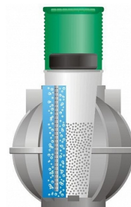
Биофильтр и аэратор
